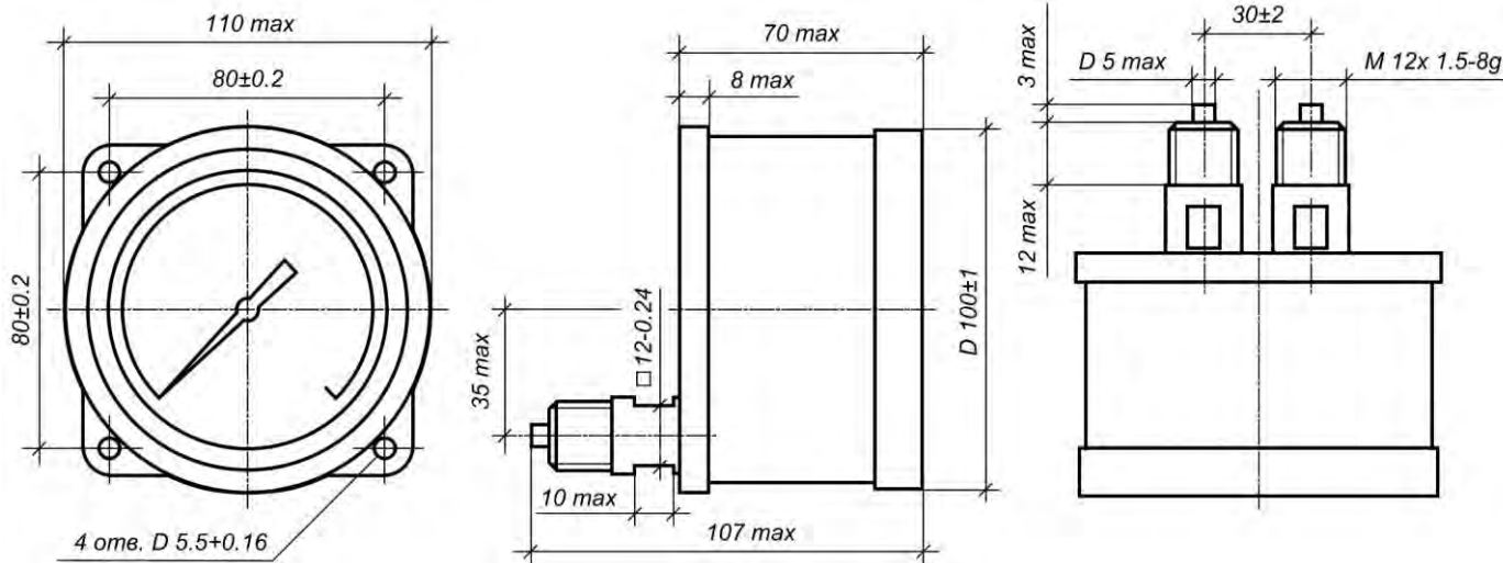
МП-2 - осевое расположение штуцера с задним фланцем
